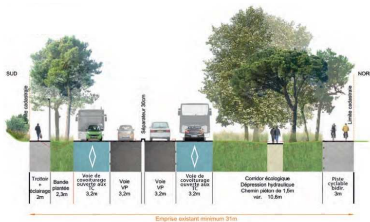
Profil en travers à Bordeaux Aéroport. © Bordeaux Métropole.
